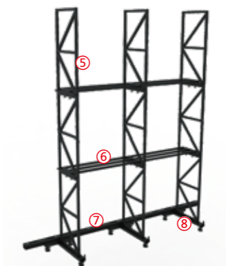
全装结构 2
